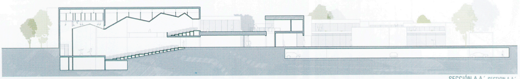
SECCIÓN A-A' SECTION A-A'
